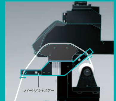
フィードアジャスター使用時のイメージ図
